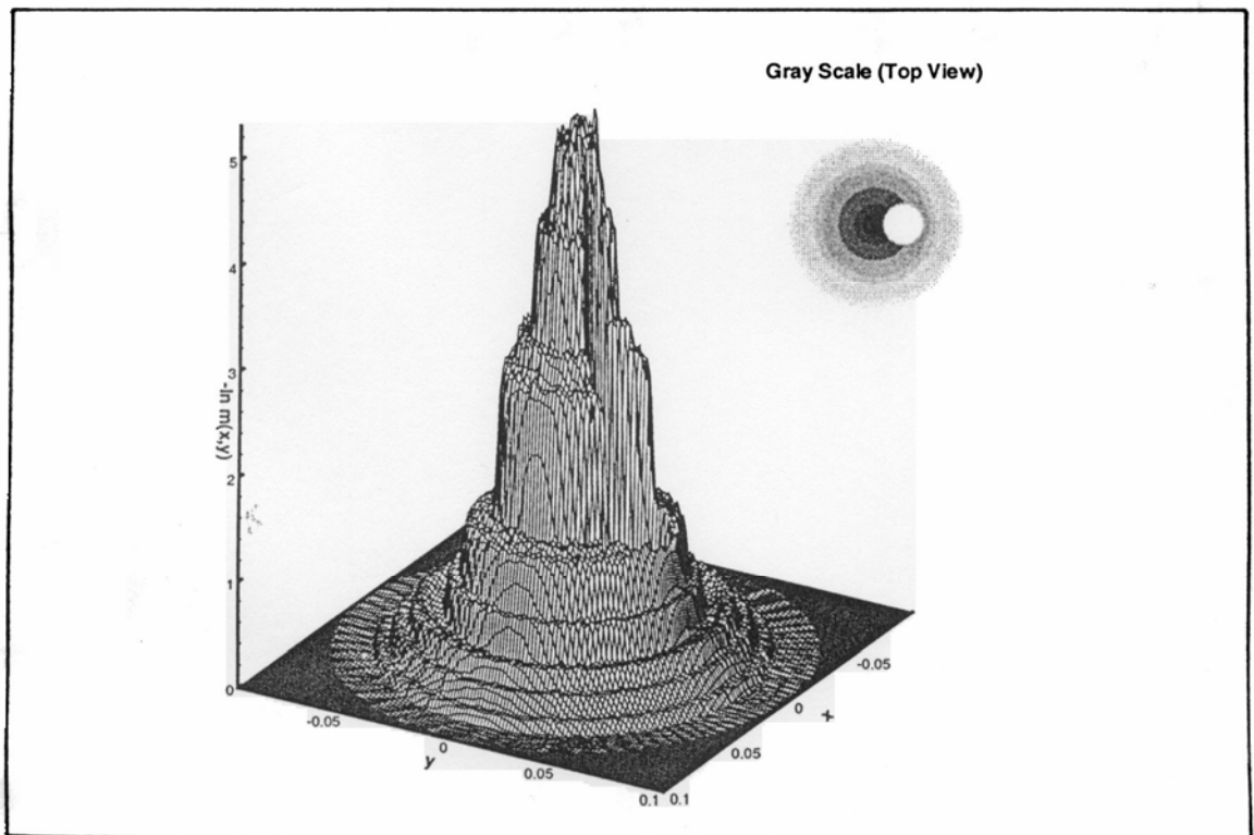
ภาพที่ 4-1 ภาพเสมือนโลคัลโมเมนต์ลำดับที่ 1 ของเปลวจำลองแบบไม่สมมาตร
